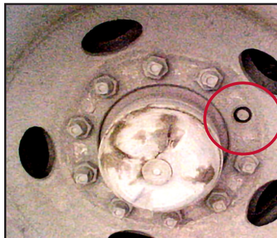
Broken stud
